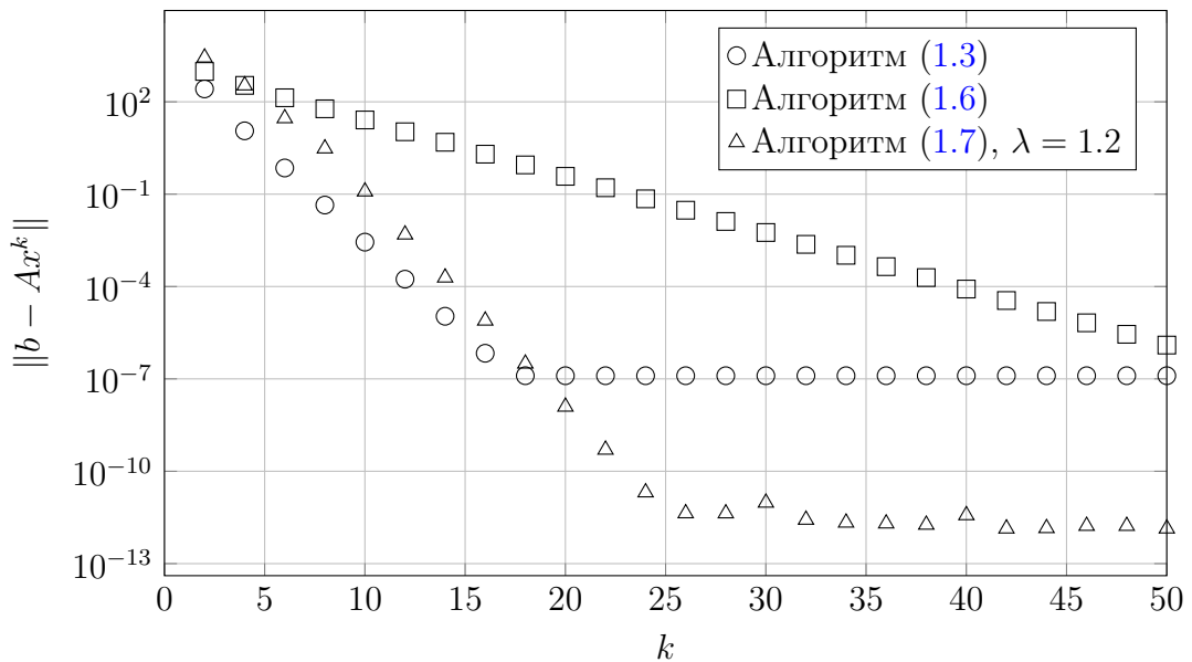
Рис. 1. Пошаговые невязки алгоритмов (1.3), (1.6), (1.7) при решении задачи согласования материального баланса, содержащей 136 уравнений и 327 неизвестных.
