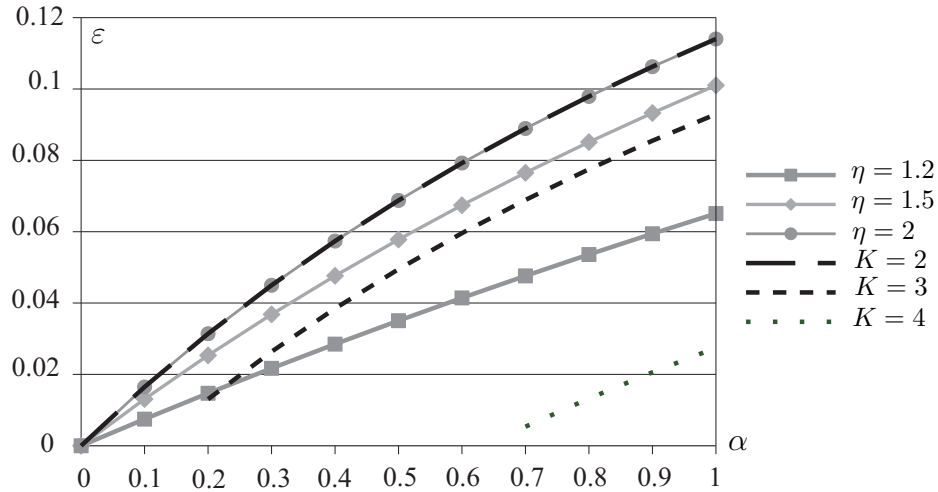
Максимальное \varepsilon , удовлетворяющее условиям теоремы 3, как функция от \alpha .
